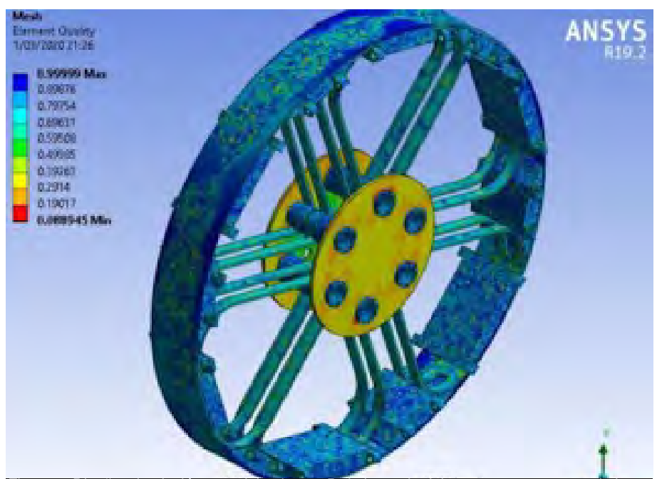
Figura 7. Diseño, simulación y modelamiento 3D de la rueda del rover con programas de ingeniería
