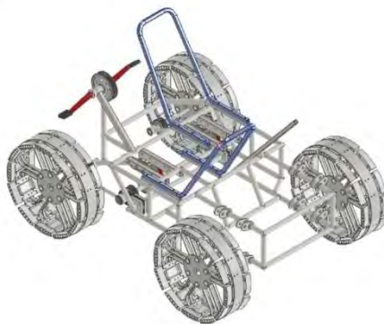
Figura 2. Diseño UNI del rover para la exploración espacial en la Luna y Marte Ref. HERC 2020 de la NASA
