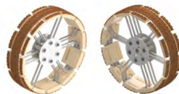
Figura 4. Diseño innovador de la rueda del rover premiada por la NASA.
